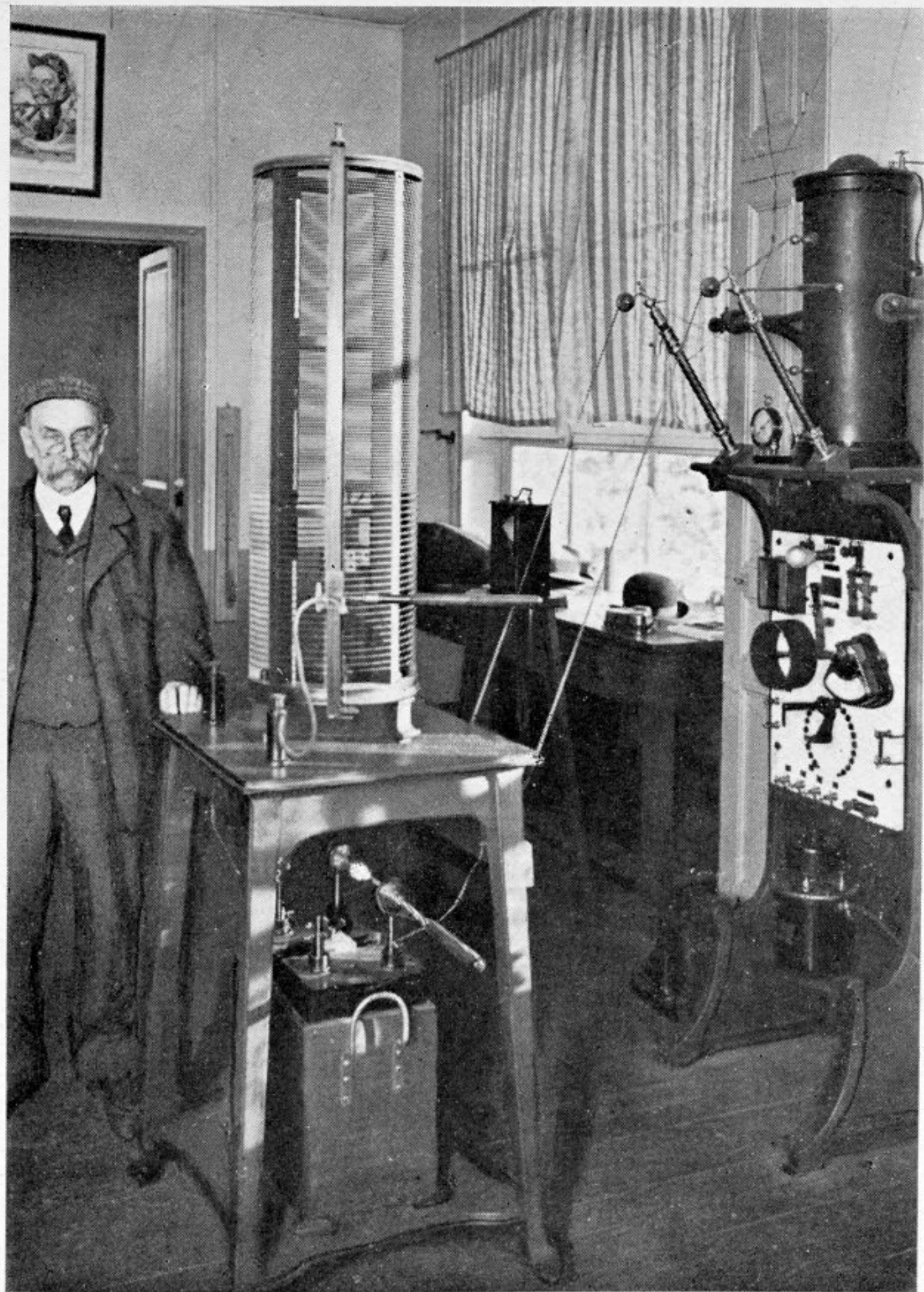
D'Arsonval essaie sur son générateur le résonateur de Oudin pour la production des courants de haute fréquence, de tension. (Laboratoire d'Arsonval.)
