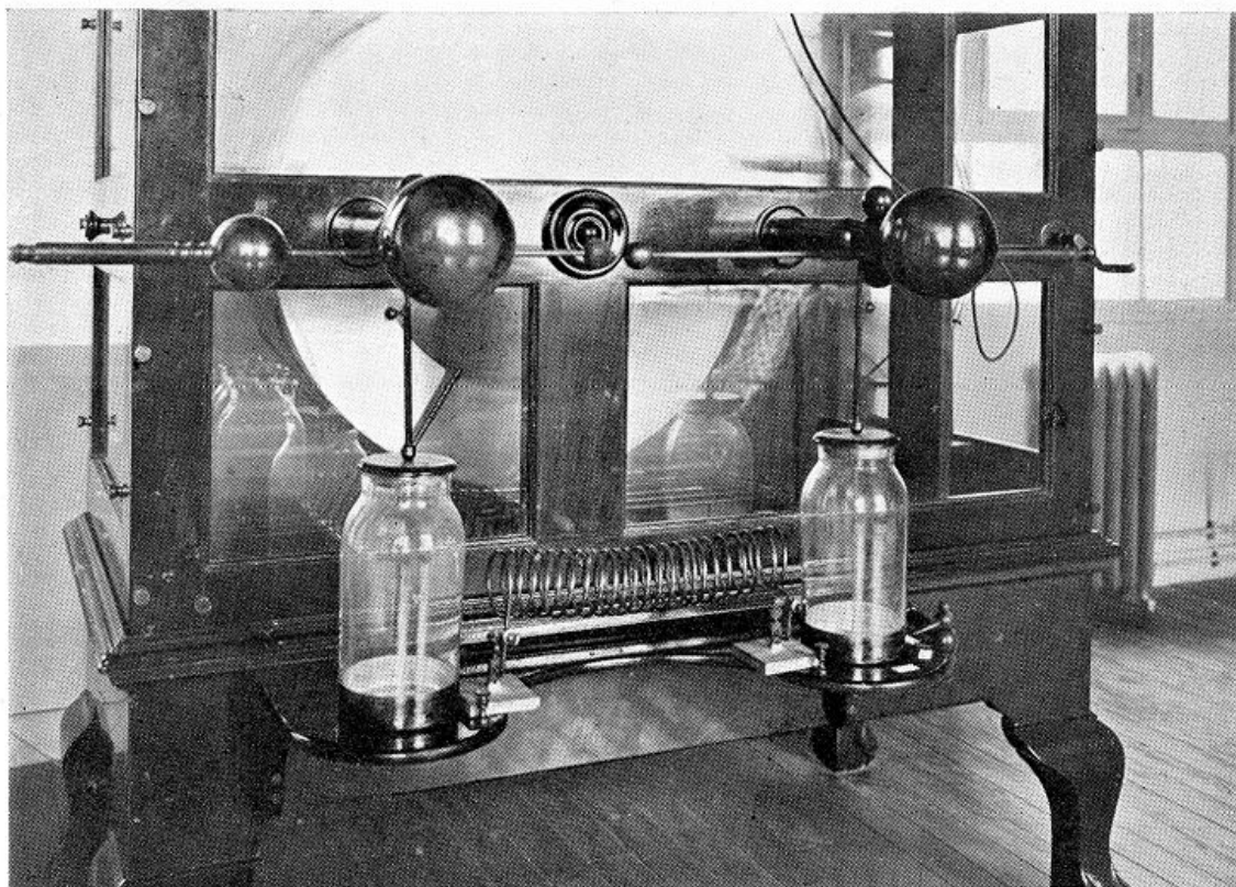
Machine statique pourvue du montage d'Arsonval pour produire les courants de haute fréquence (1892). (Laboratoire d'Arsonval.)
