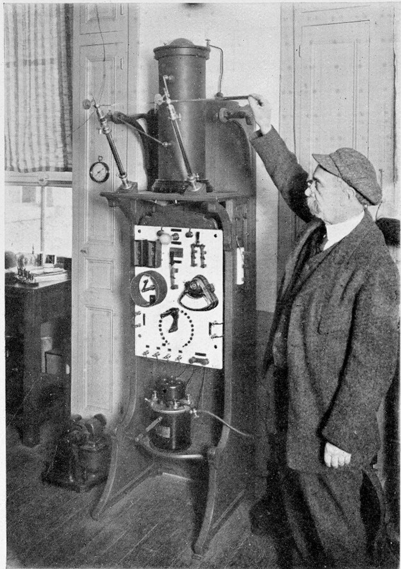
D'Arsonval règle l'éclateur d'un générateur de haute tension utilisé pour la production des courants de haute fréquence. (Laboratoire d'Arsonval.)
