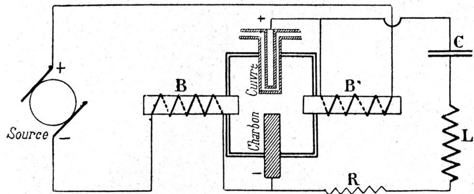
Fig. 18. — Dispositif pour produire l'arc de Poulsen.
