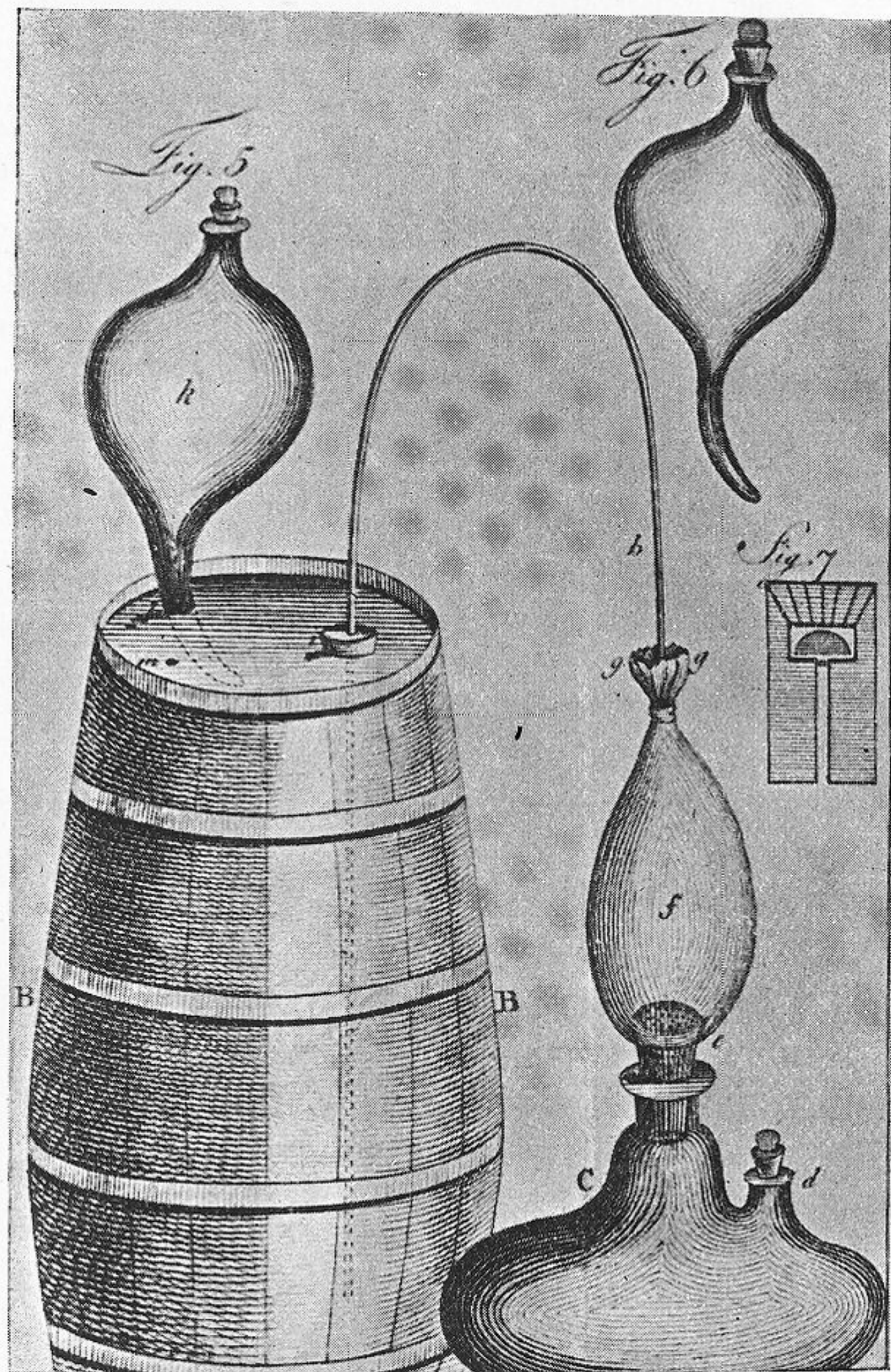
FIG. 8. Henry's Apparatus.
