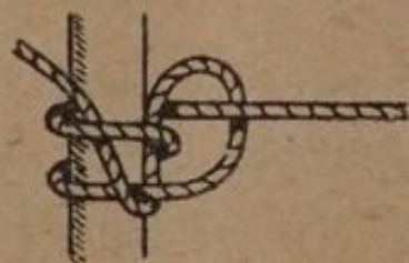
HALLIARD HITCH
