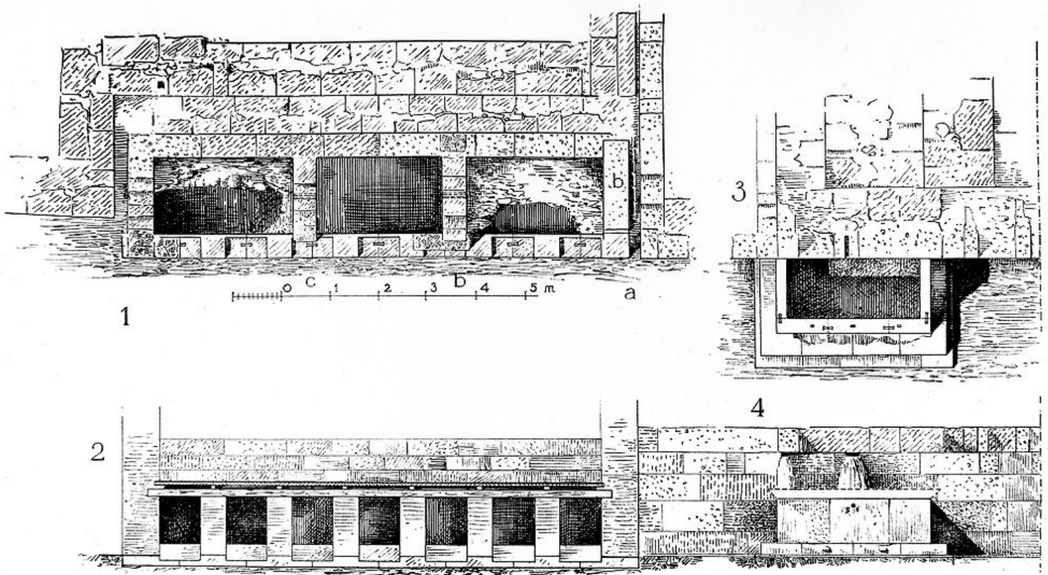
Brunnenkammern und Westbrunnen Grundriß und Ansicht (hellenistischer Zustand)
