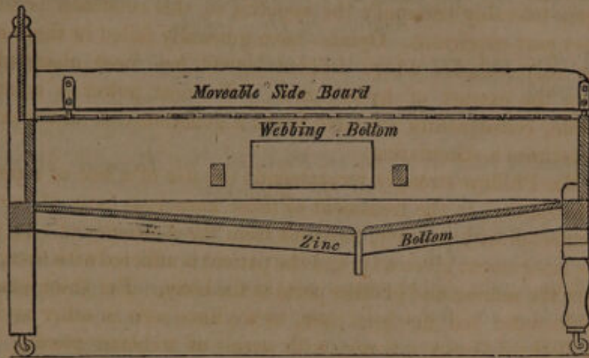
LONGITUDINAL SECTION.
