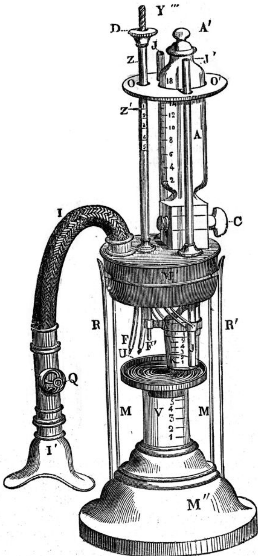
FIG. 12. — Anesthésimètre de Duroy (appareil monté).
