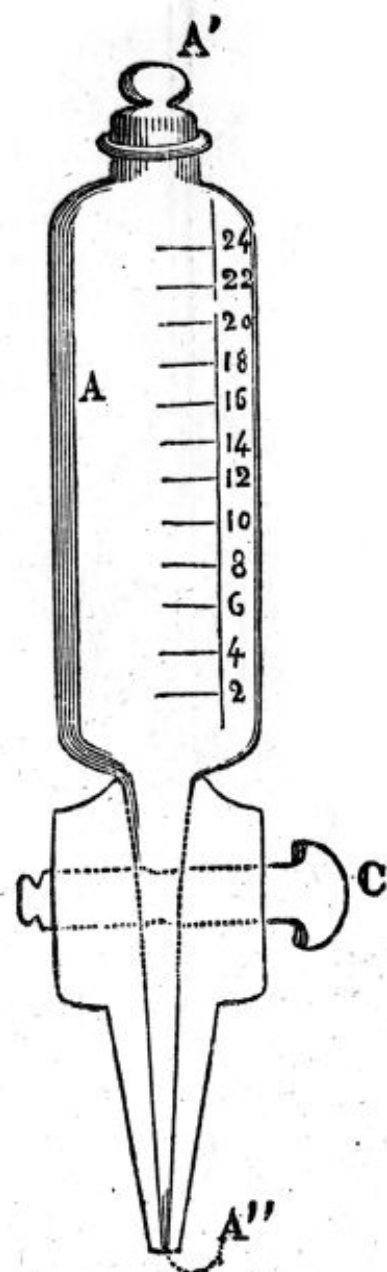
FIG. 13. — Anesthésimètre de Duroy (réservoir à déplacement).
