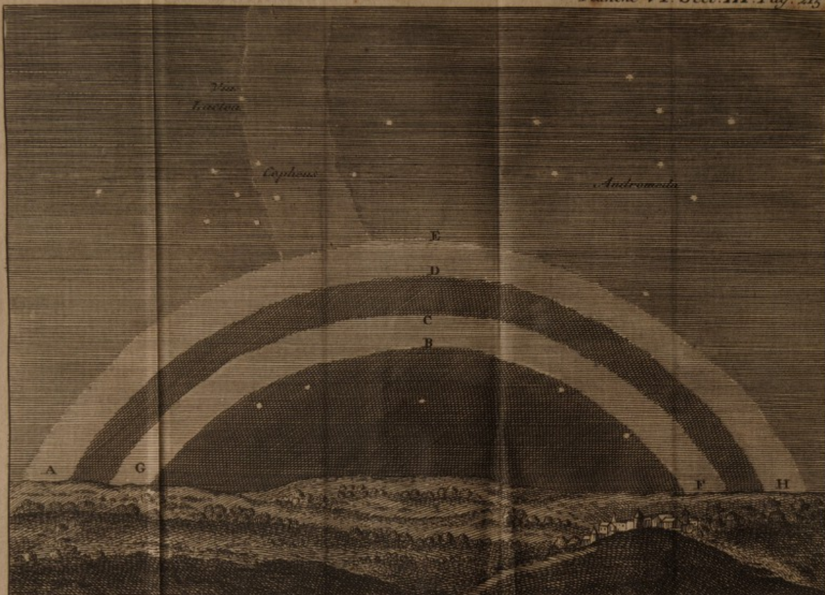
Fig. XI. Aurore Boreale vue à Giessen le 17 me Fevrier 1721. d'après la figure qui en fut donnée dans les Actes de Lipsic, dépouillée des rayons et jets de Lumiere.
