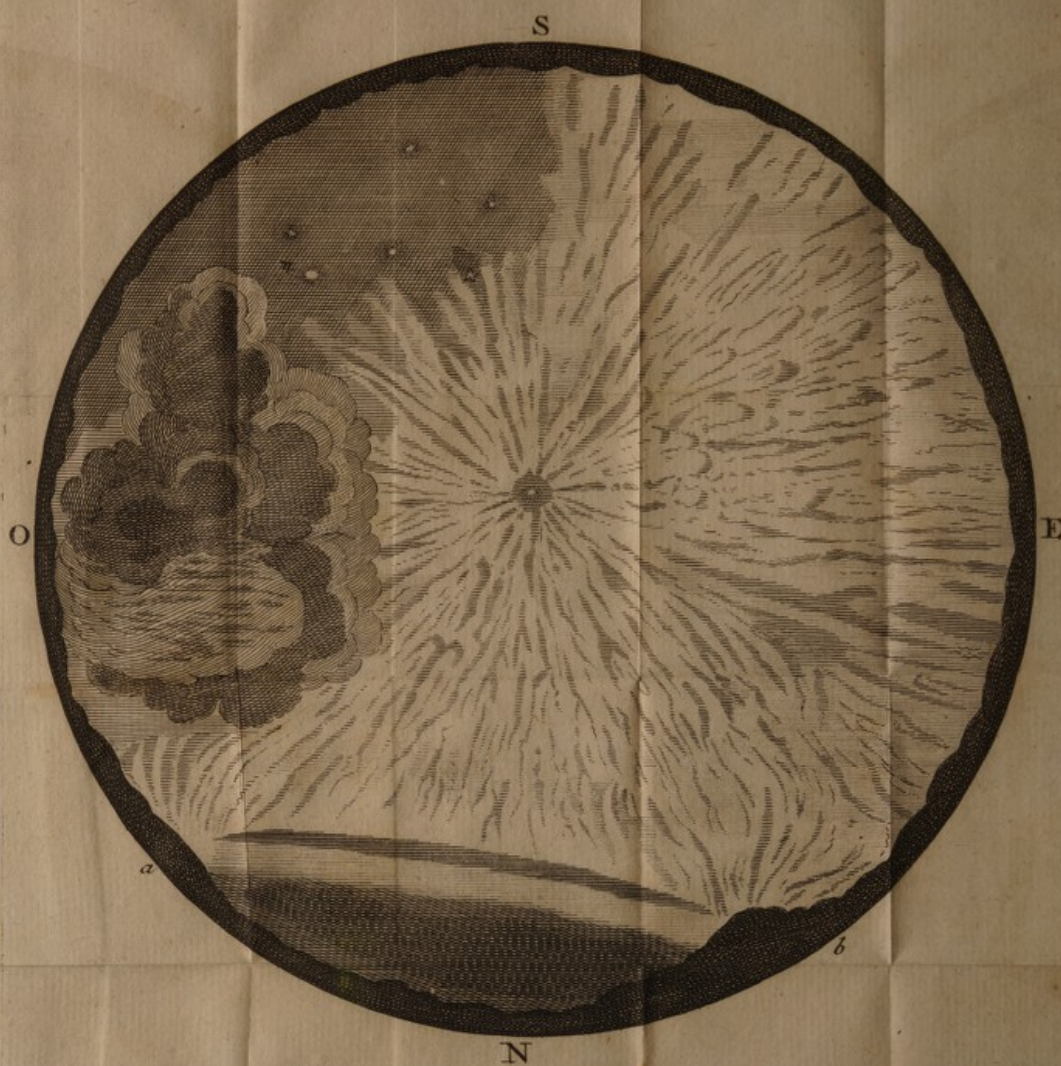
Fig. XVII. Aurore Boreale du 19 me Octobre 1726. telle qu'elle parut dans tout l'Hemisphère Superieur du Ciel, vers les 8 heures du Soir; à Breuillepont, Diocese d'Évreux, 15 ou 16 Lieues à l'Occident de Paris.
