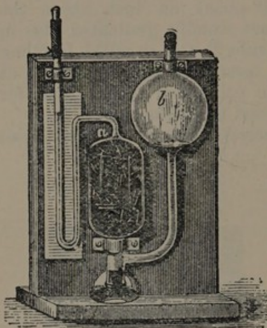
FIG. 5.—Phosphorus Pipette.
