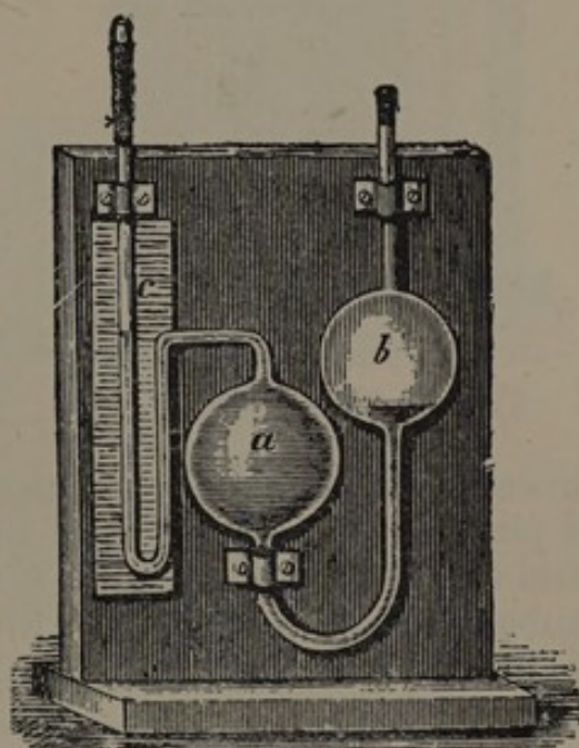
FIG. 4.—Gas Pipette.
