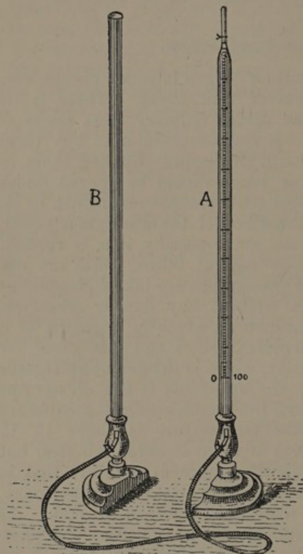
FIG. 3.—Hempel's Apparatus.
