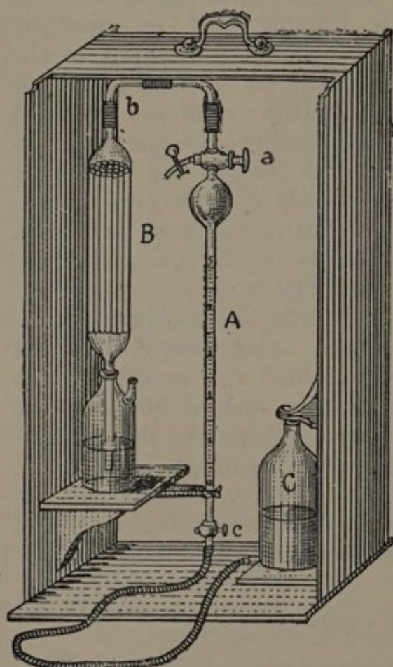
FIG. 14.—Winkler's Apparatus.
