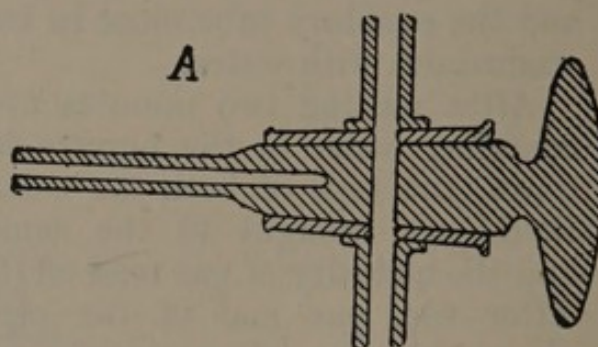
FIG. 12.—Tap.
