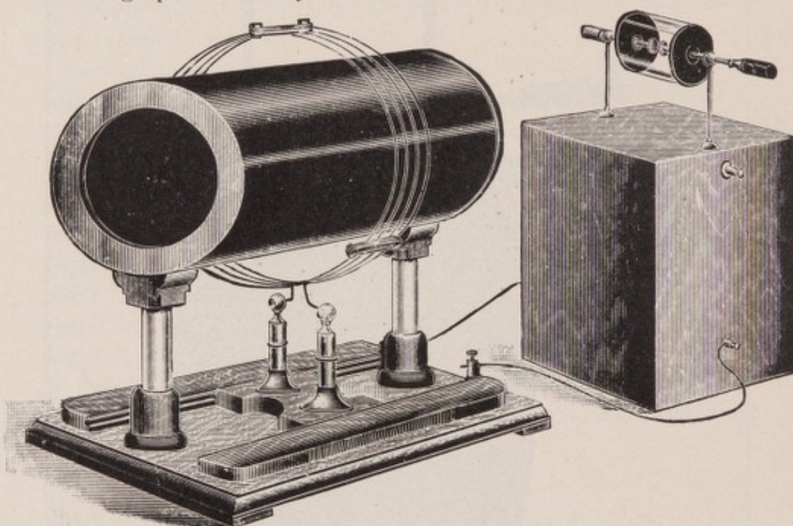
FIG. 45.—Gaiffe’s Bipolar Resonator.
