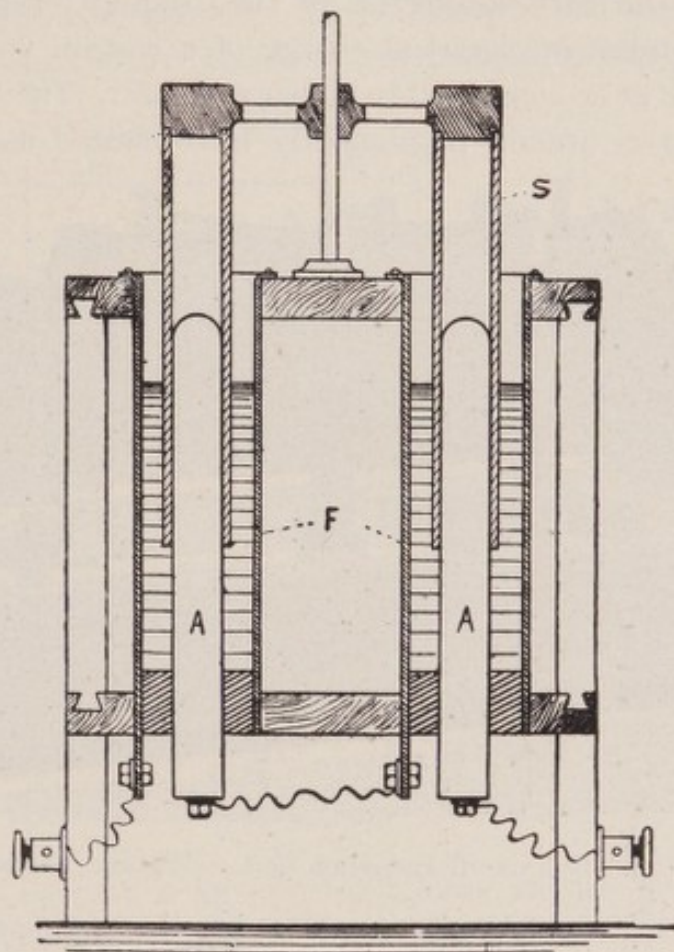
FIG. 32.—Nodon Valve, or Rectifier. (Williams.)
