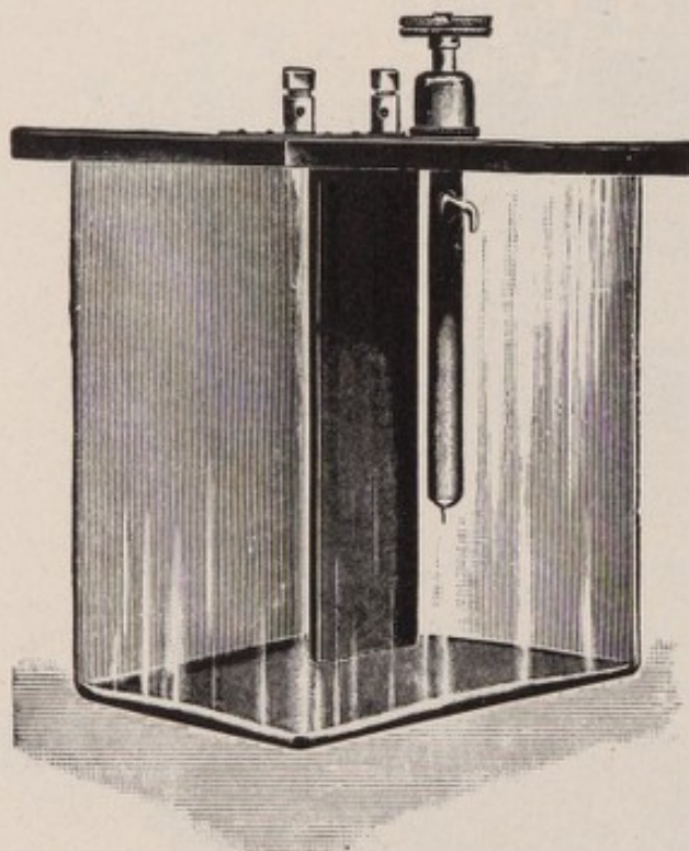
FIG. 38.—Wehnelt Interrupter. (Williams.)
