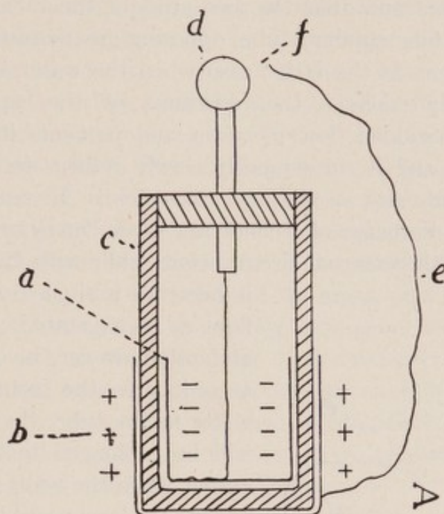
FIG. 23.—Leyden Jar, or Condenser.
