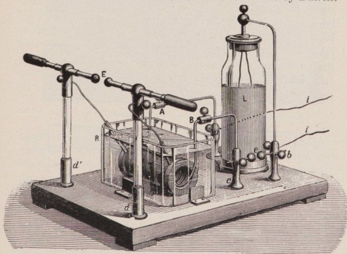
FIG. 4.—Miniature Tesla Apparatus. (E. Ducretet.)
