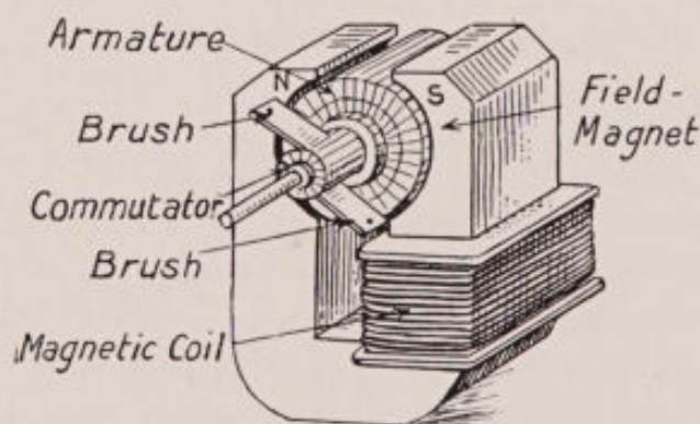
FIG. 26.—Plan of dynamo.
