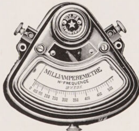
FIG. 56.—Hot wire milliampère meter.
