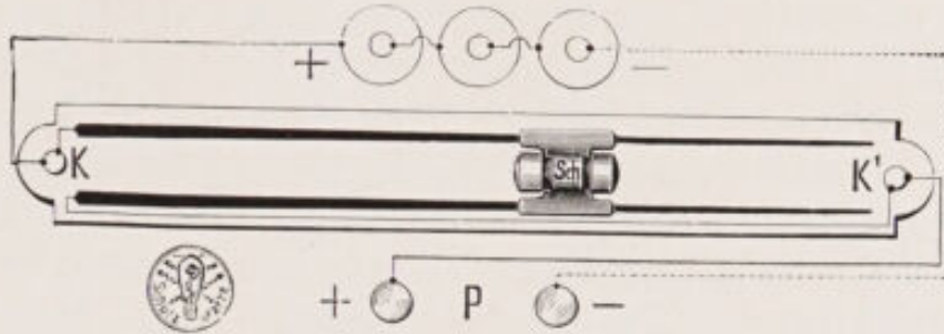
FIG. 39.—Graphite rheostat.
