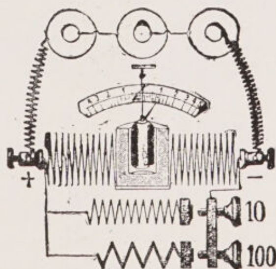
FIG. 37.—Plan of shunt.
