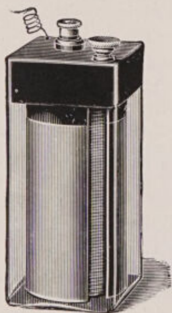
FIG. 7.—Wet Leclanché cell.
