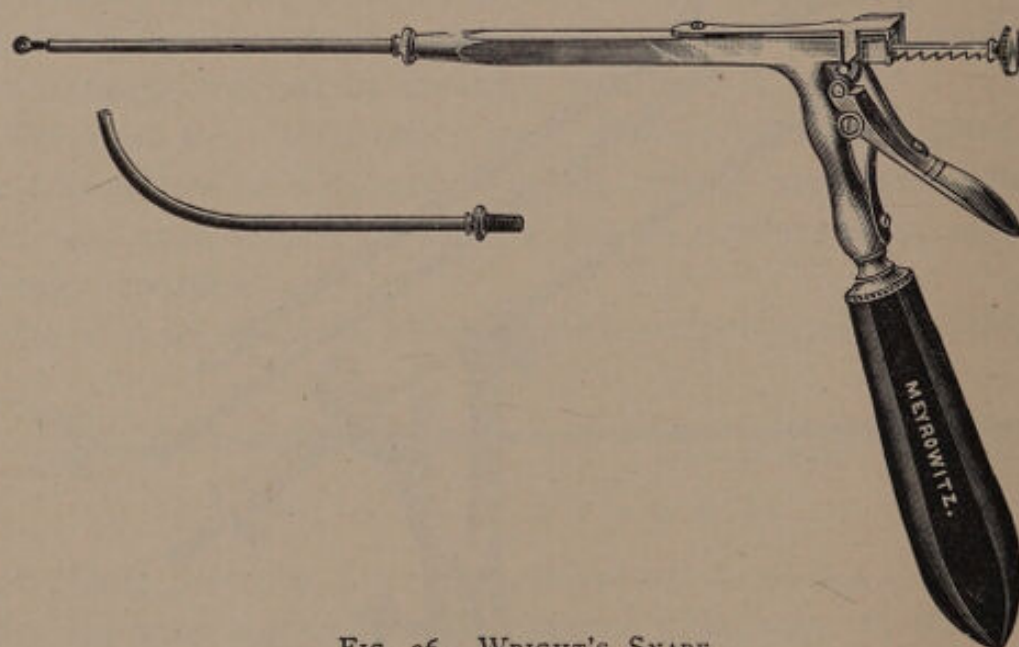
FIG. 26. WRIGHT'S SNARE.
