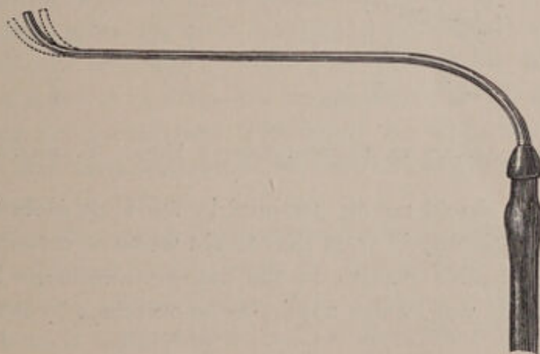
FIG. 39. HARTMANN'S CANULA.
