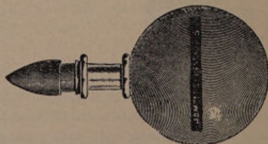
FIG. 22. NASAL SYRINGE.
