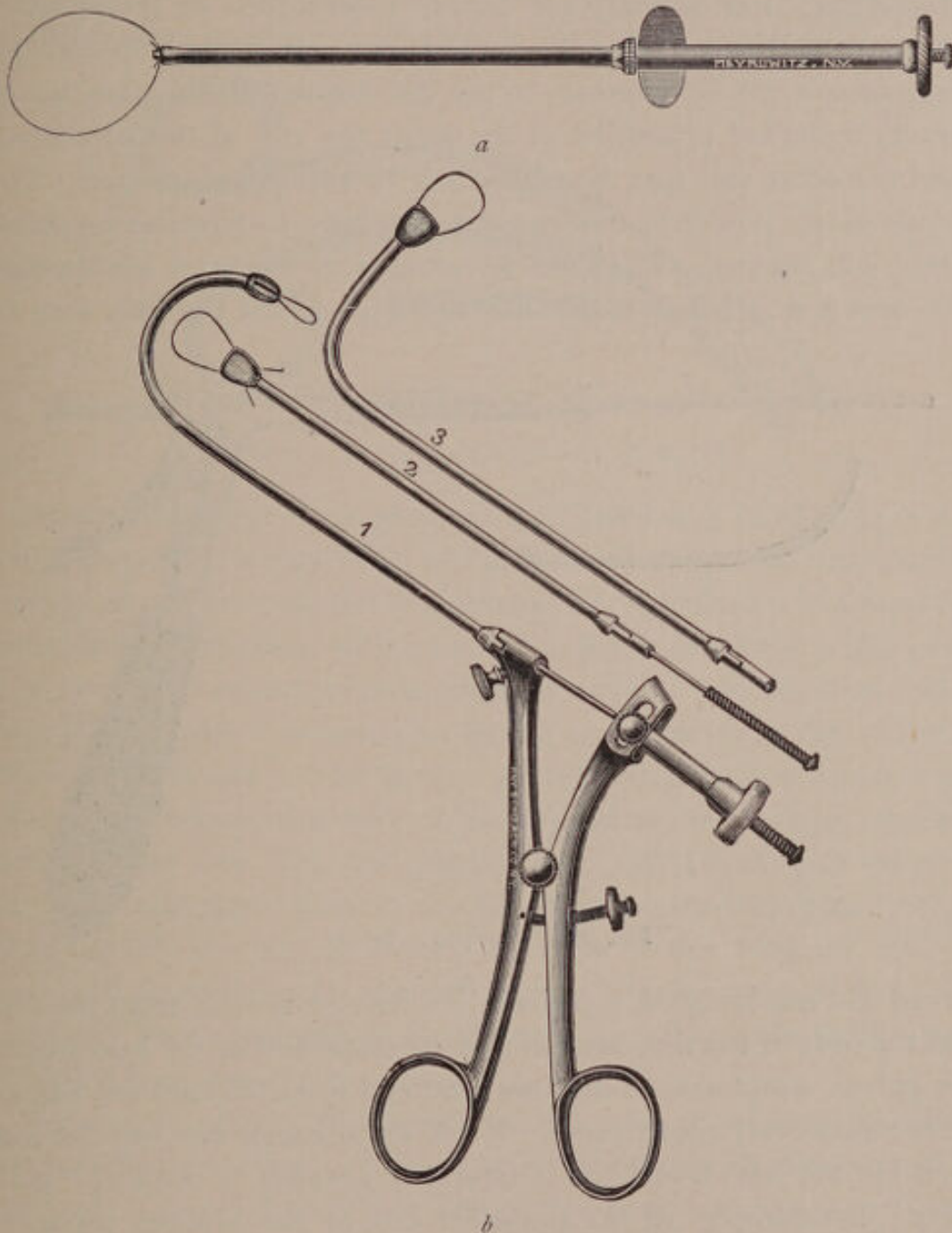
FIG. 25. SAJOUS' SNARES.
