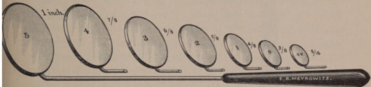
FIG. 112. LARYNGEAL MIRRORS.
