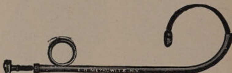
FIG. 67. BELLOCQ'S CANULA.
