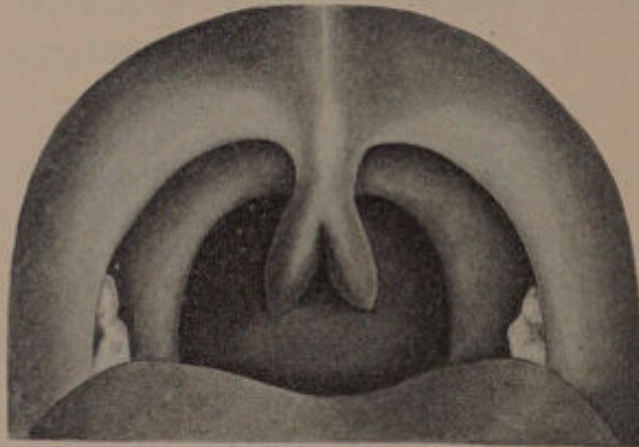
FIG. 78. BIFID UVULA.
