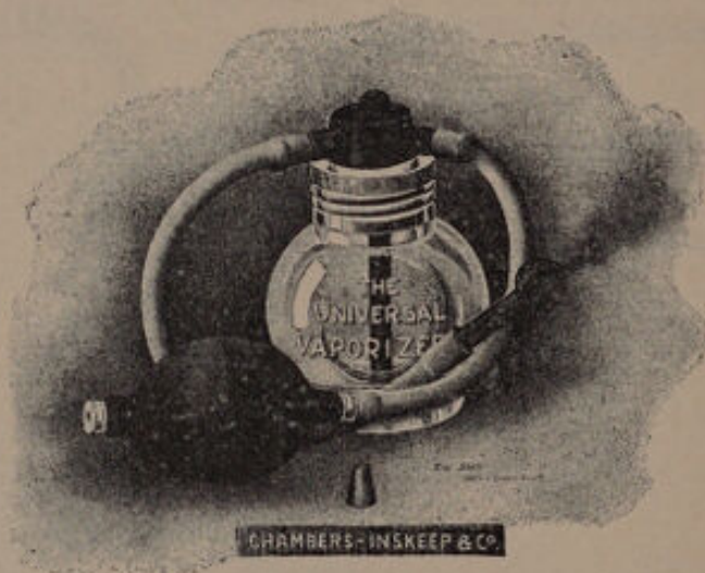
FIG. 16. UNIVERSAL VAPORIZER.
