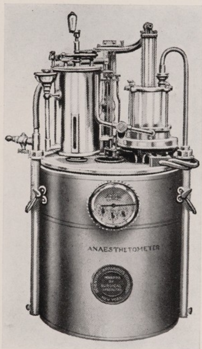
FIG. 82.—Anæsthetometer (Connell).
