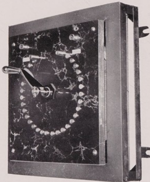
Fig. 29. Twenty-nine button rheostat.
