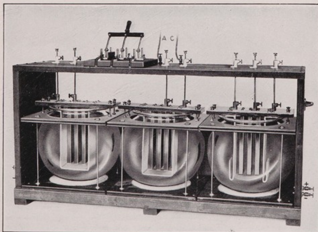
Fig. 28. Three-cell rectifier.
