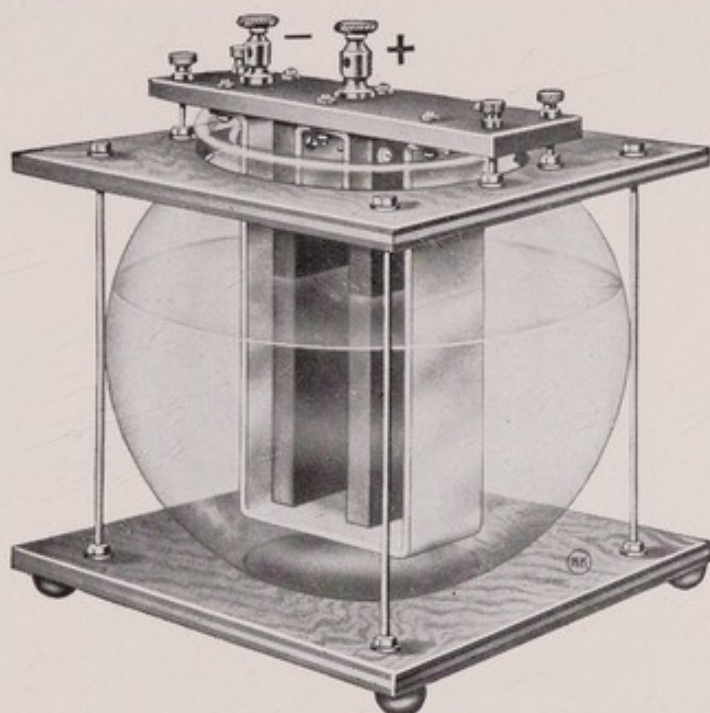
Fig. 27. One-cell rectifier.
