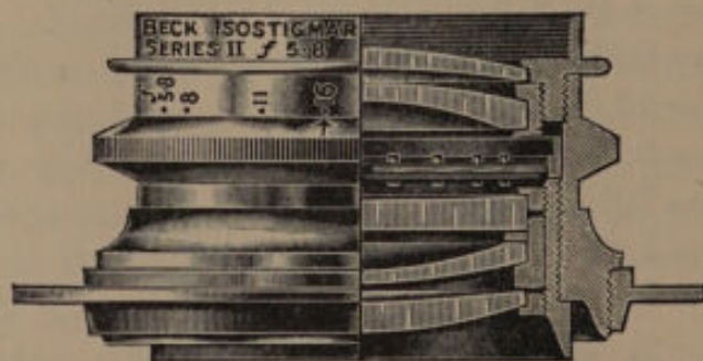
FIG. 93.—Beck's Isostigmat.
