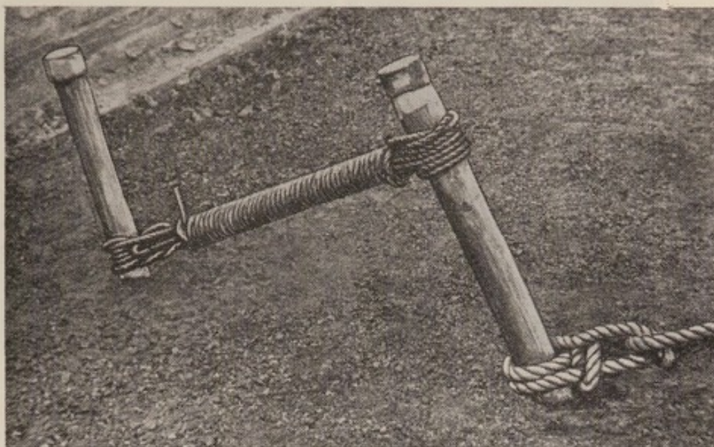
Fig. 85 (d). A 1 and 1 picket
