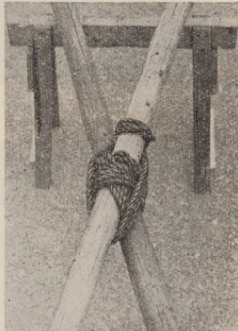
Fig. 66 (d). Diagonal lashing
