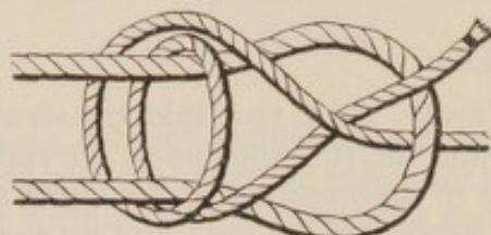
Fig. 57. Double sheet bend
