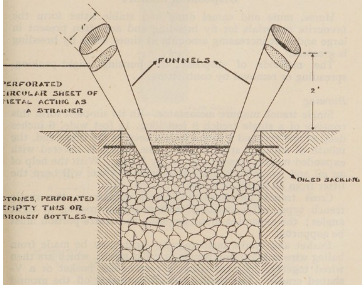
FIG. 28.—Funnel Urine Pit.
