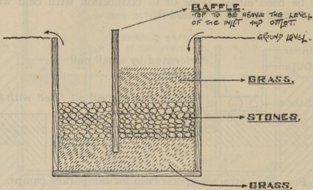
FIG. 33A.—Strainer trap.
