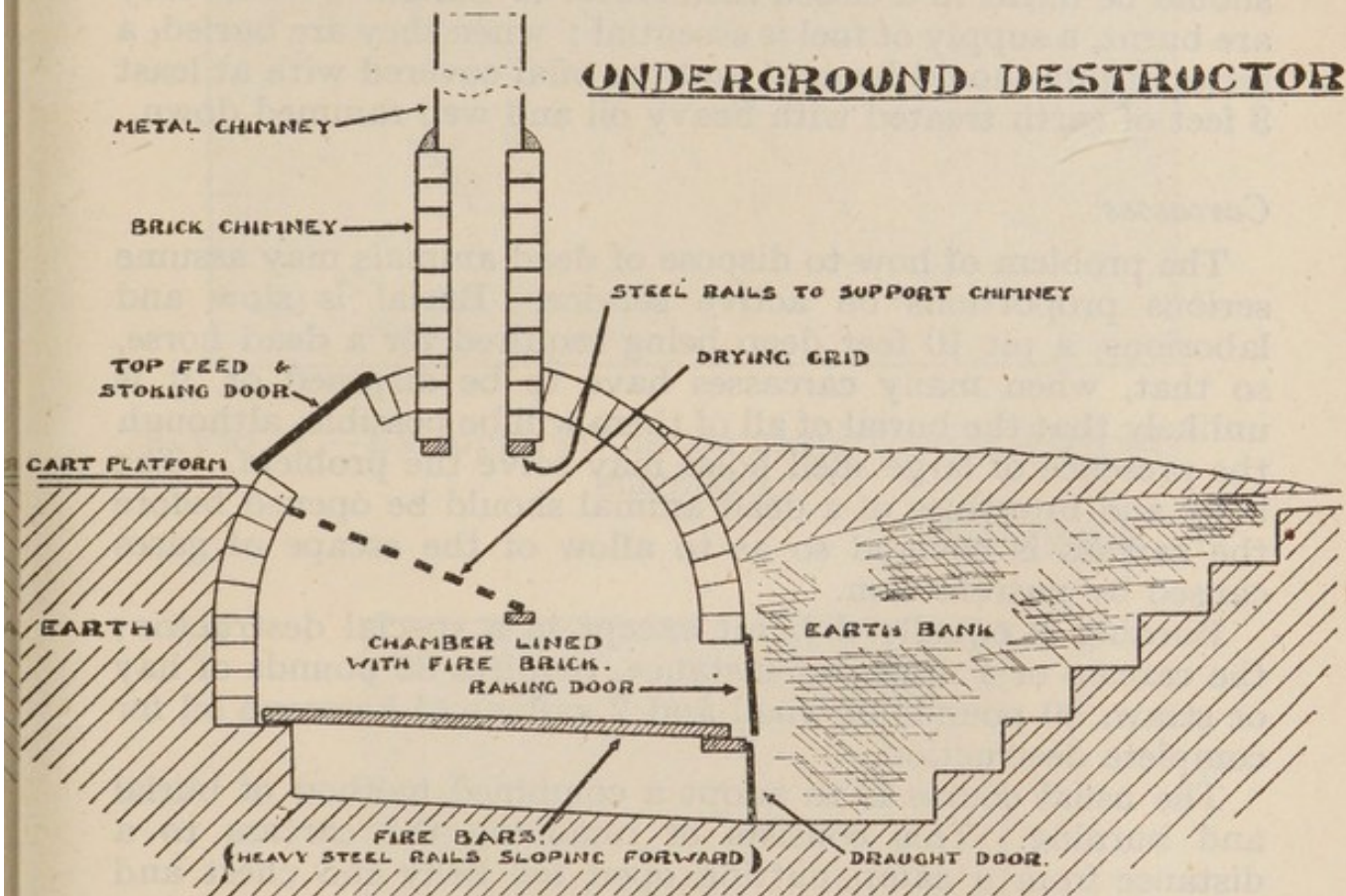
FIG. 44.—Underground destructor.
