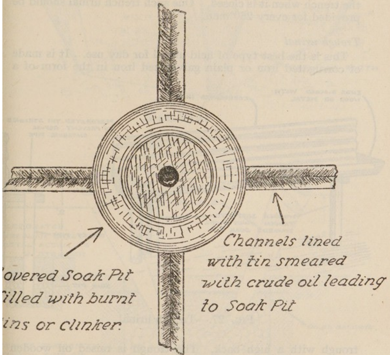
FIG. 26.—Abdast.
