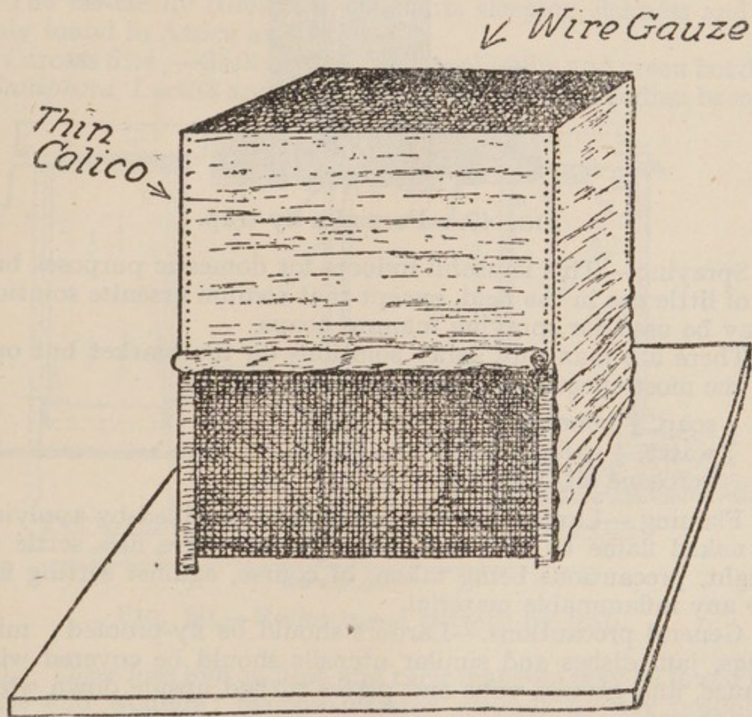
FIG. 48.—Box fly trap.
