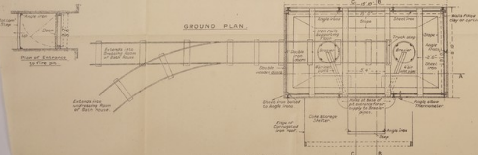
FIG. 60.—Or's bat. Hot air disinfestor.
