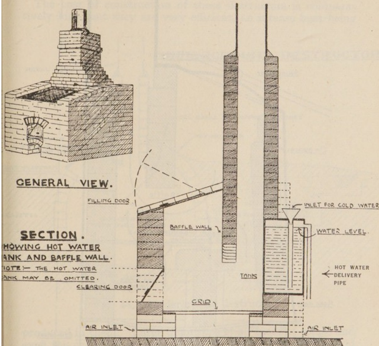
FIG. 42.—Bailleul incinerator.
