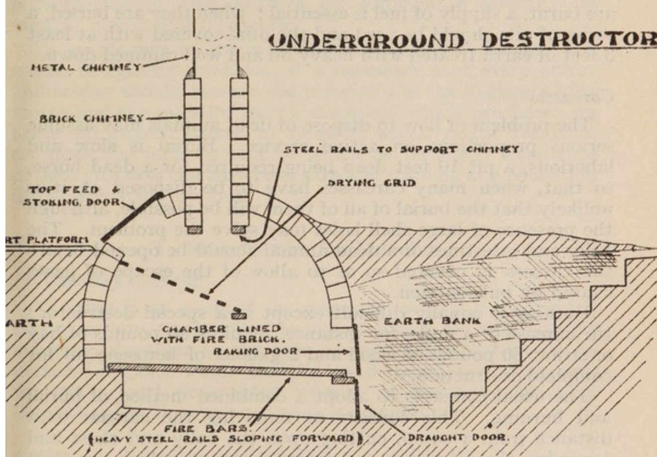
FIG. 44.—Underground destructor
