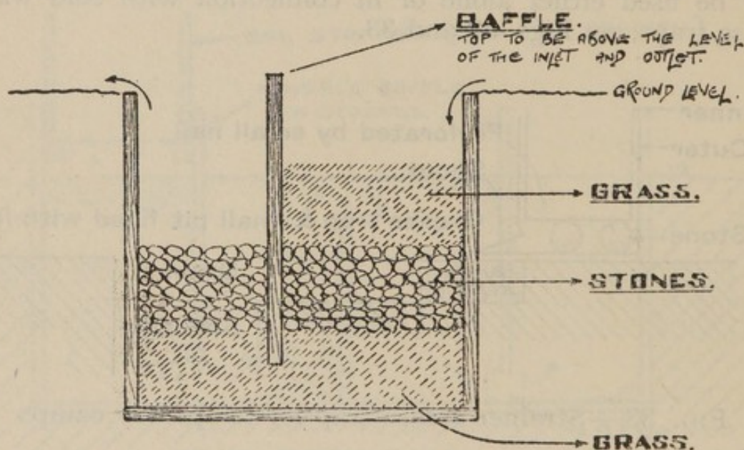
FIG. 33A.—Strainer trap.
