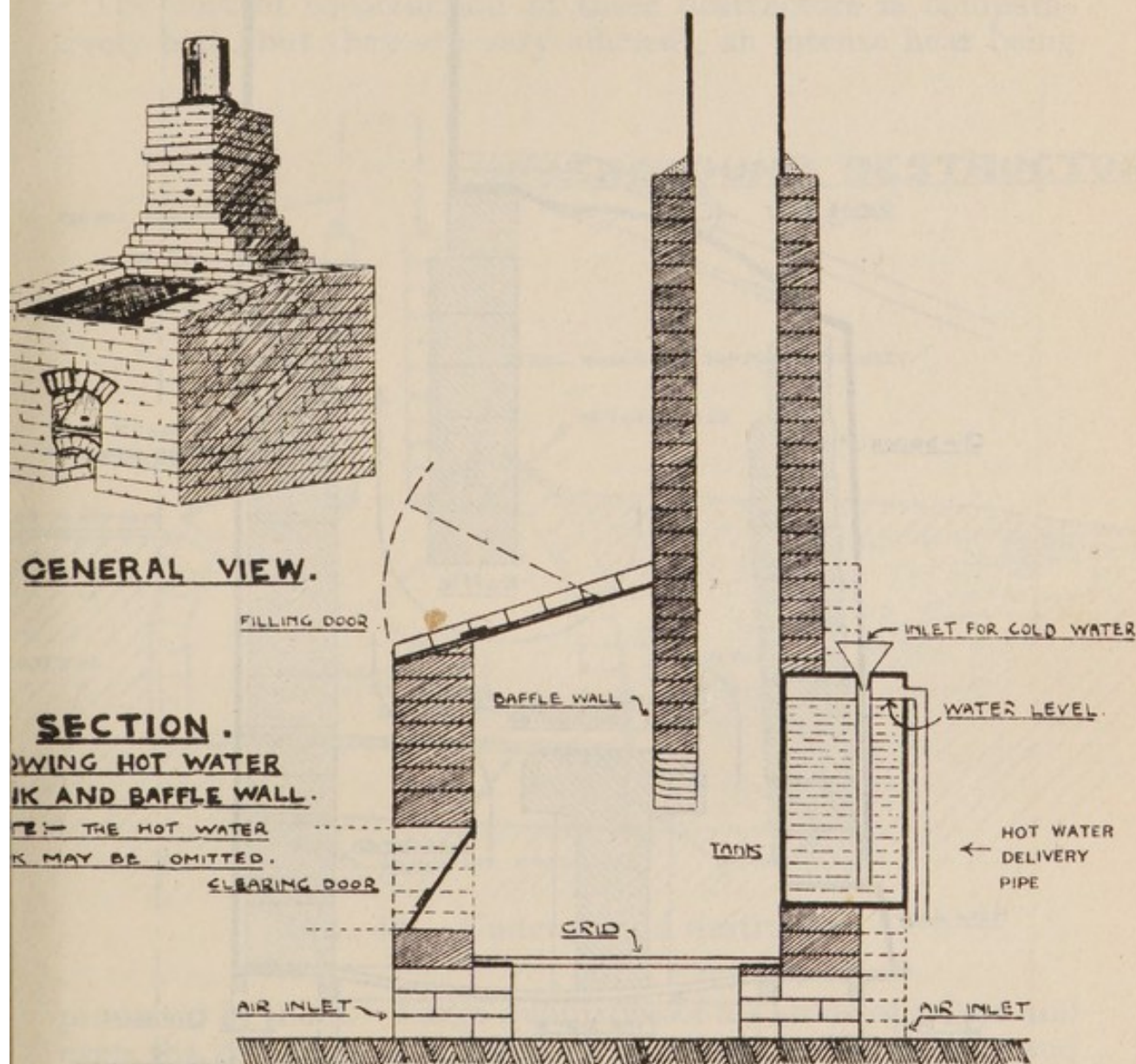
FIG. 42.—Bailleul incinerator.
