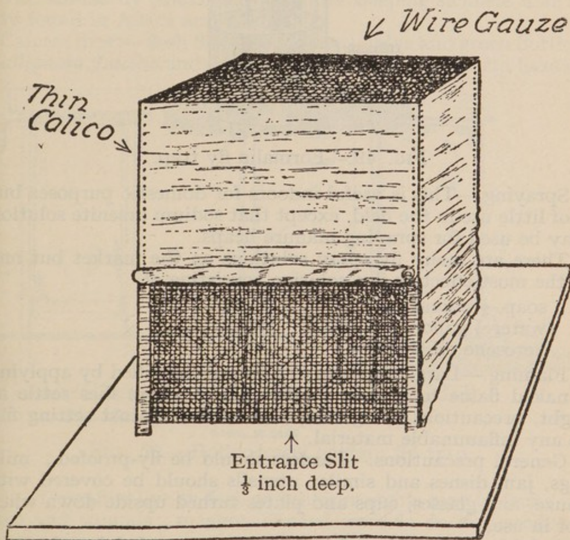
FIG. 48.—Box fly trap.
