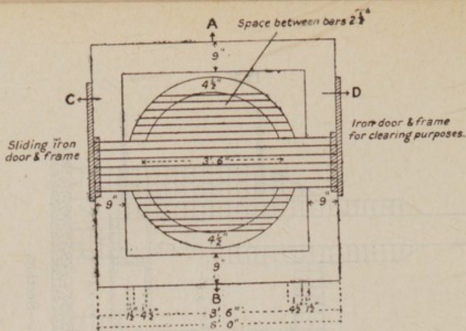
FIG. 35.—Plan.
