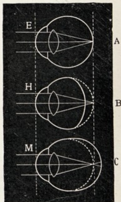
FIG. 259. — A, EMME- TROPIA. B, HYPERME- TROPIA. C, MYOPIA.
