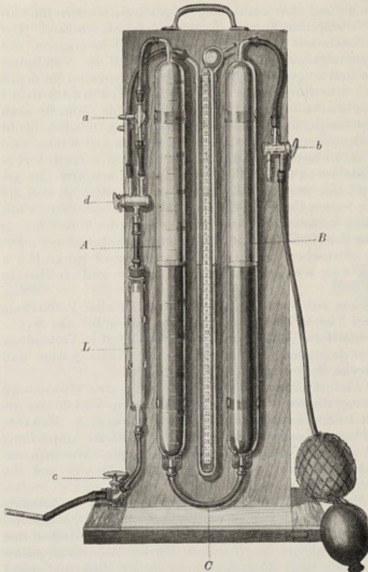
Abb. 19. Pneumothoraxapparat nach v. MURALT. Vorderansicht.
