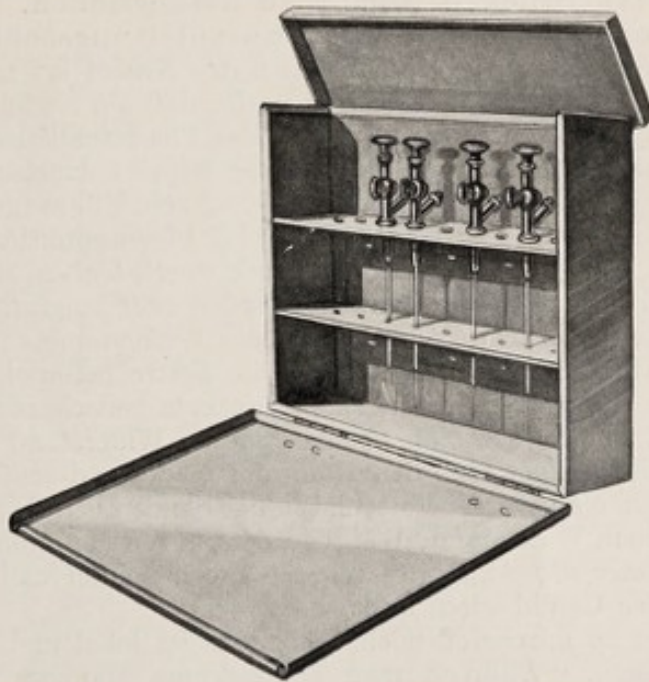
Abb. 21. Metallhülse für Sterilisation und Aufbewahrung der Pneumothoraxnadeln.
