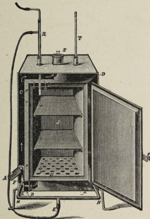
Fig. 10.—Hot-air sterilizer.
