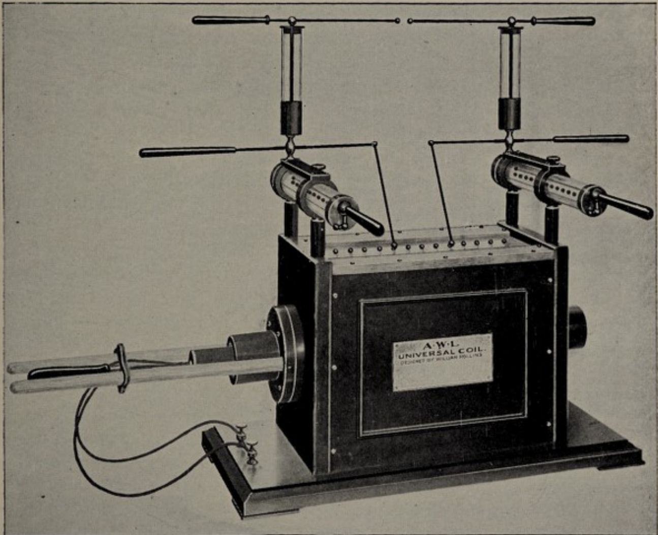
FIG. 21. A. W. L. universal coil. 43 centimetres. (Rollins.)
