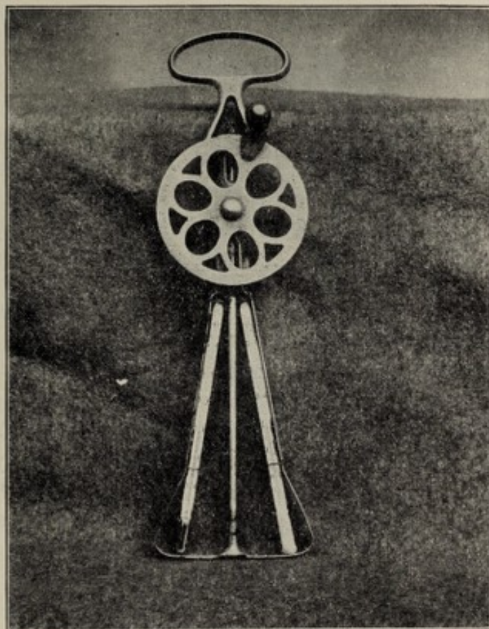
Fig. 6. Cog psychrometer.
