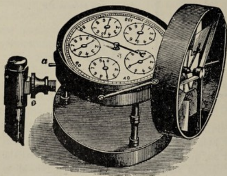
Fig. 23. Simple anemometer.
