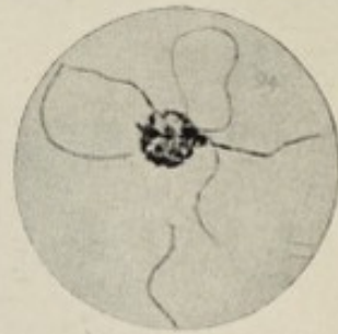
Fig. 132.—Microgametocyte, showing flagella (Koch).
