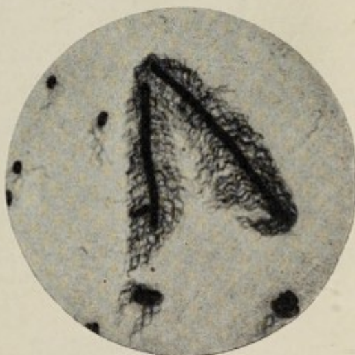
Fig. 101.— B. proteus , showing flagella (Migula).
