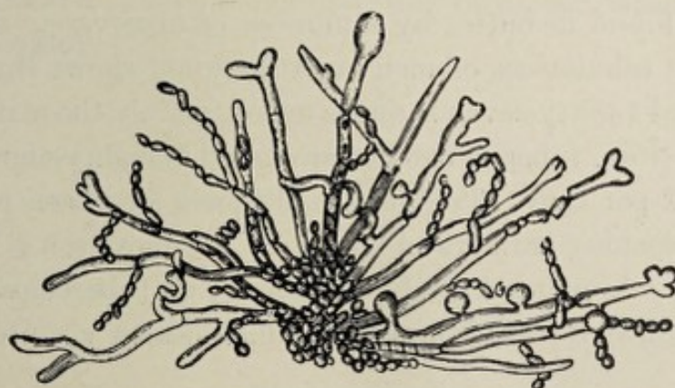
Fig. 145.— Oidium lactis colony on gelatin (Conn).
