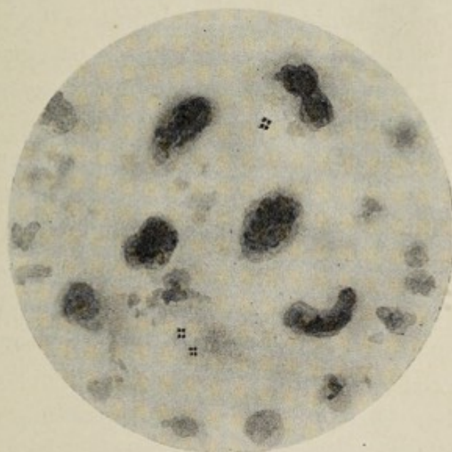
Fig. 46.— Micrococcus tetragenus from peritoneal pus (Bythell).
