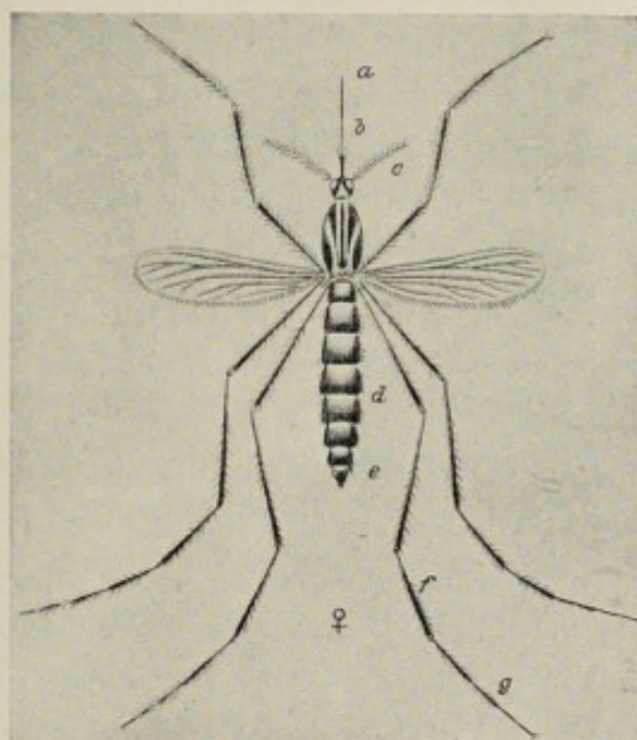
Fig. 162.— Stegomyia calopus , female. \times 8 . a , Proboscis; b , palpi; c , antenna; d , femur; e , tibia; f , metatarsus; g , tarsus (Otto).
