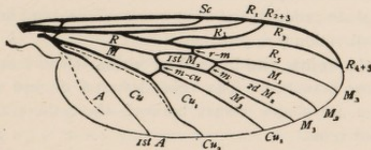
FIG. 2.—Wing of Rhyphus .
