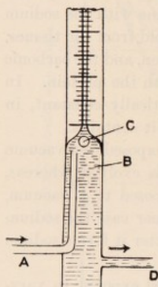
FIG. 124. —Krogh's tonometer.
