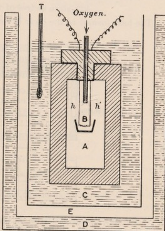
FIG. 156.—Bomb calorimeter.
