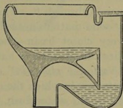
FIG. 16.—WASH-OUT WATER-CLOSET.
