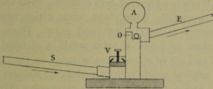
FIG. 8.—HYDRAULIC RAM.
