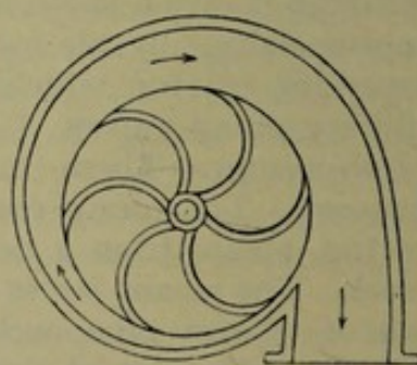
FIG. 7.—CENTRIFUGAL PUMP.
