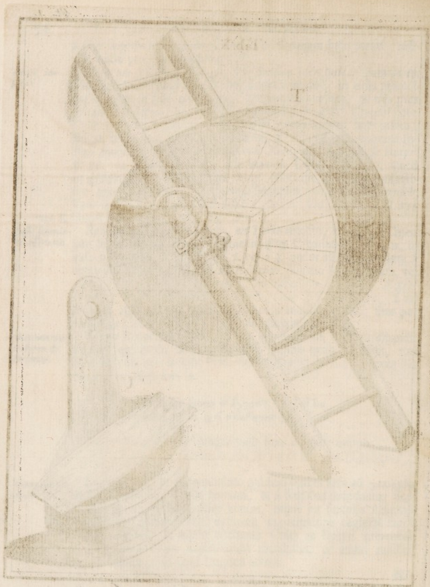
Fig. 1. Wasser-Rad mit einem Schöpfen.
