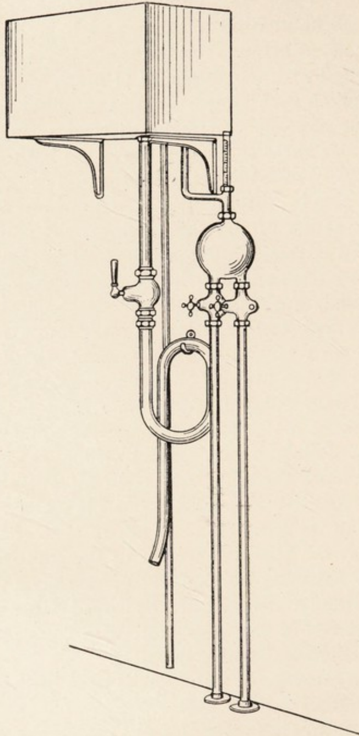
FIG. 4.—LOW-PRESSURE DOUCHE.
