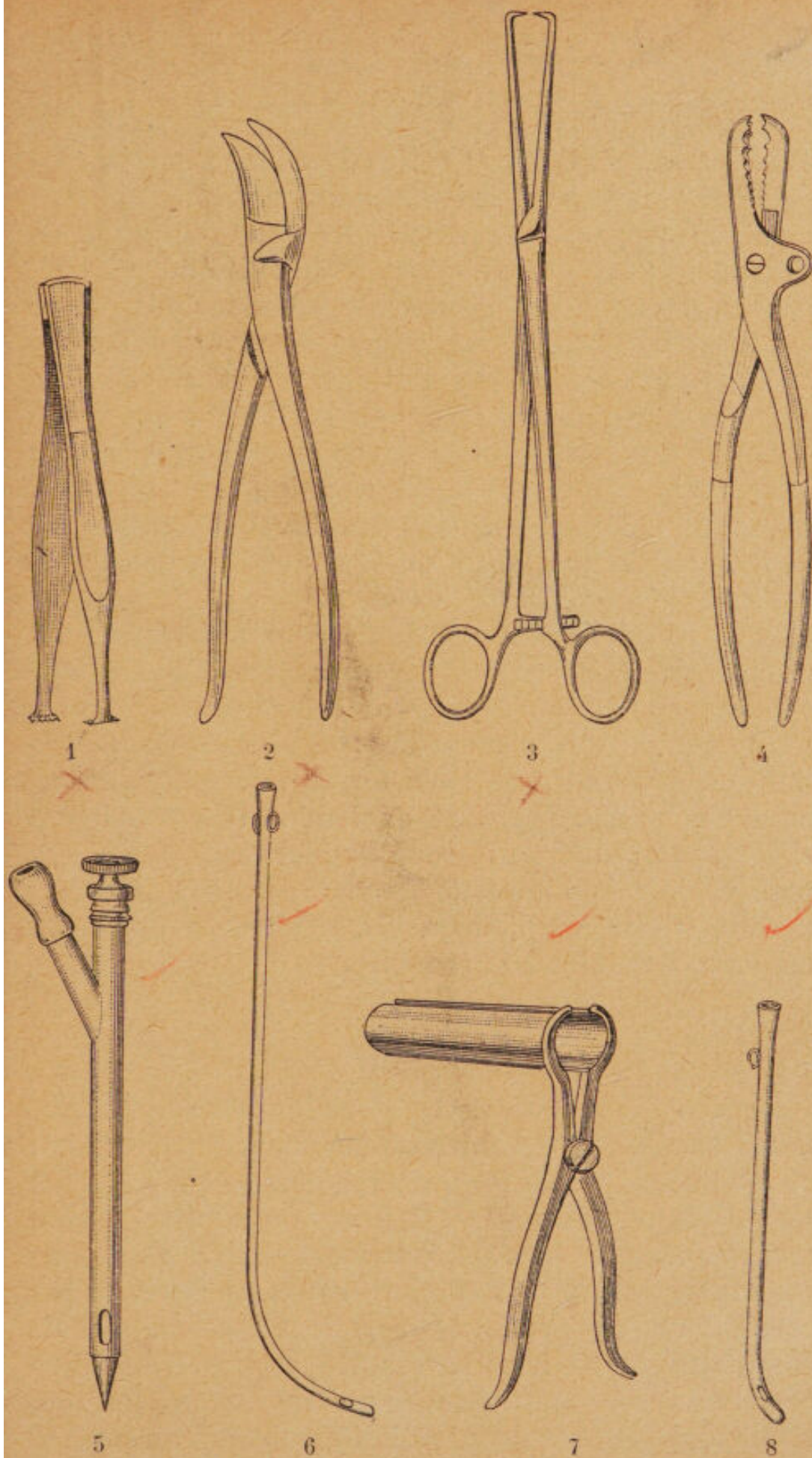
FIG. 13 à 20. — Instruments modernes correspondants à ceux de la figure 5 à 12 (1, pince à disséquer; 2, ciseaux; 3, pince à traction; 4, davier; 5, trocart à ponction; 6, sonde uréthrale pour homme; 7, spéculum dilateur; 8, sonde uréthrale pour femme).
