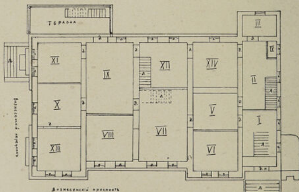
Планъ верхняго этажа дома Н. Н. Ипатьева.
