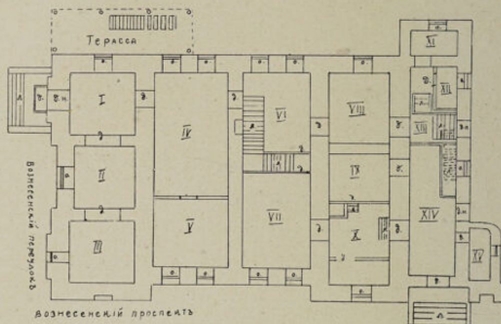
Планъ нижняго этажа дома Н. Н. Ипатьева.
