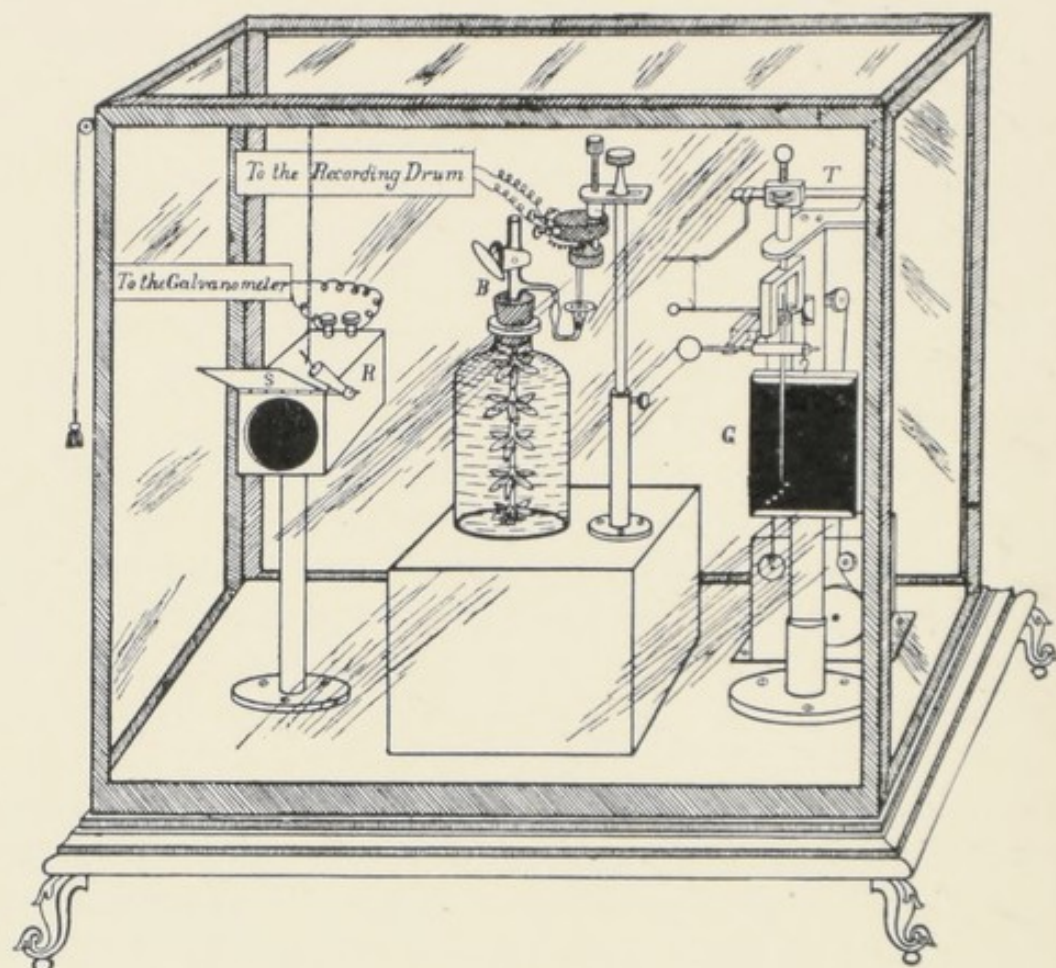
FIG. 43. The Complete Apparatus
