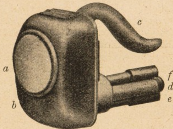
Fig. 5 a. Quarz-Wasserlampe nach Prof. Kromayer. \frac{1}{3} der natürl. Größe. a Quarzfenster. b Metallgehäuse. c Griff. d Abflußrohr. e Zuflußrohr für das Wasser. f Stromzuleitung.
