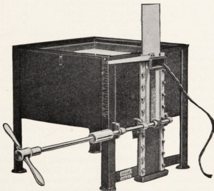
FIG. 145.—WATER PHANTOM.
