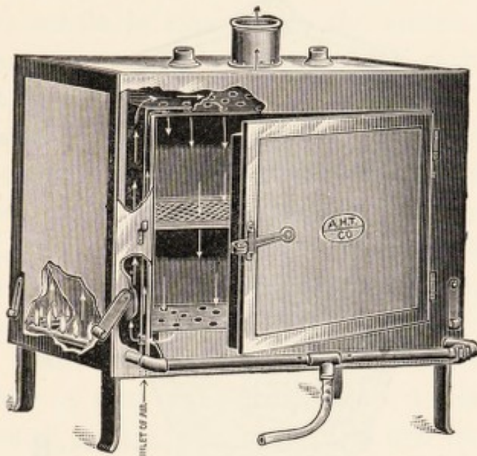
Fig. 10.—Dry heat sterilizer.
