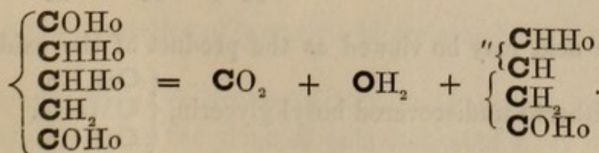
Itatartaric acid.
