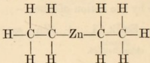
Zincic ethide.
