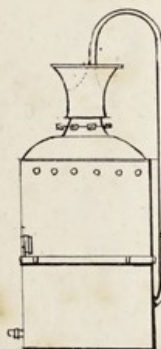
Appareil distillateur.
