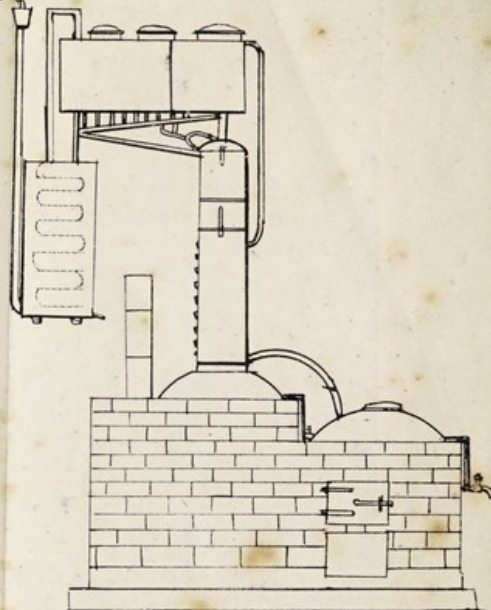
Appareil Distillateur.
