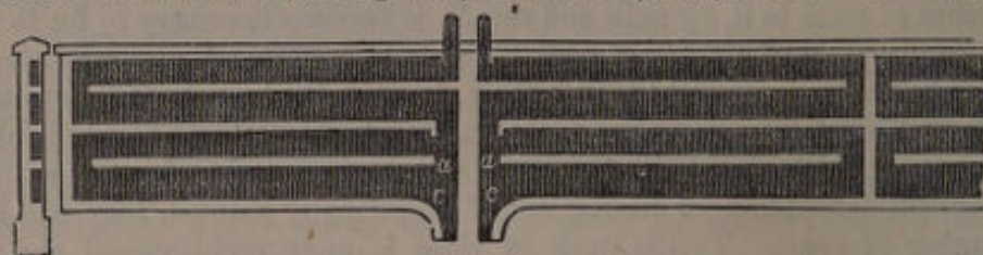
Fig. 121. Longitudinal section of a flued wall.
