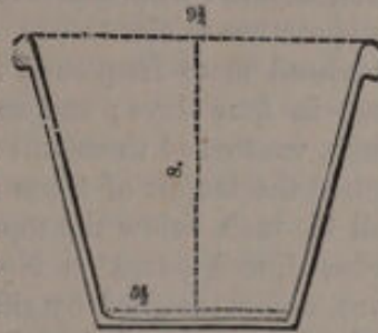
Fig. 341. A No. 16 pot.
