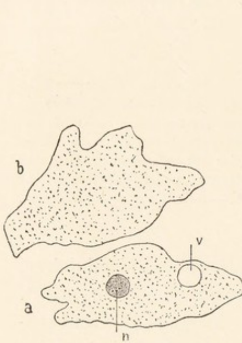
FIG. 3. — Une Amibe immédiatement après la section en deux parties. a. Moitié avec le noyau n ; b. moitié sans noyau; v . vacuole contractile. (D'après BRUNO HOFER.)
