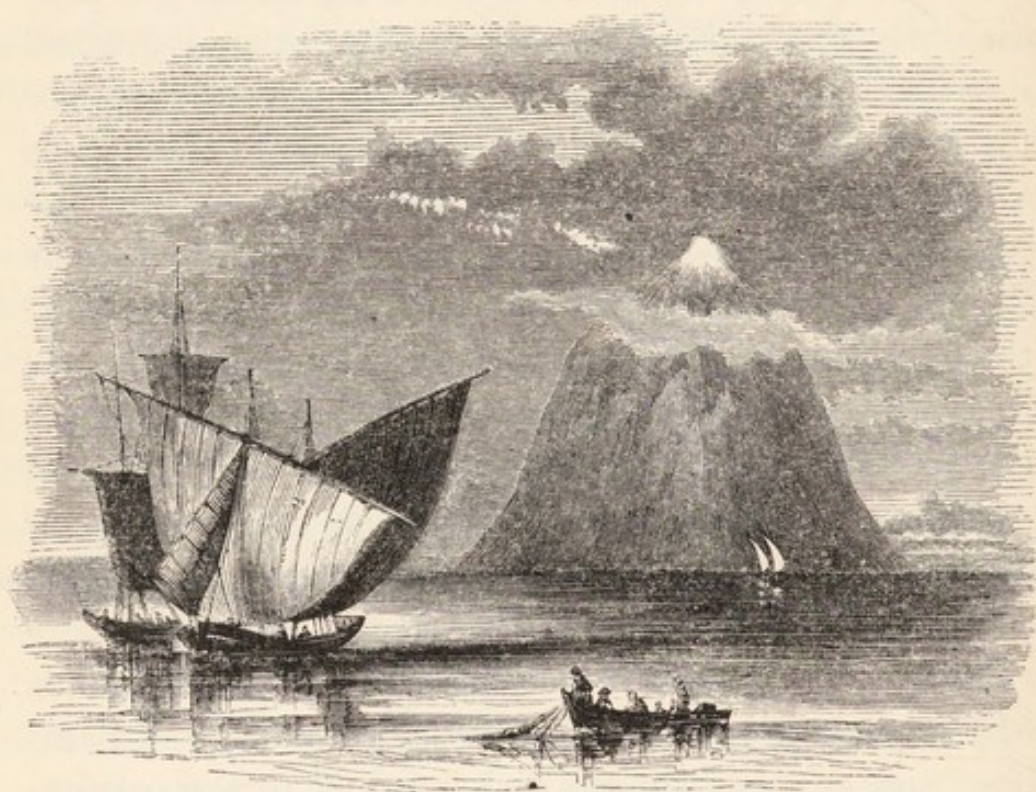
PICO.
