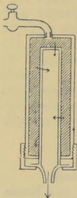
Fig. 98. PASTEUR-CHAM- BERLAND FIL- TER.
