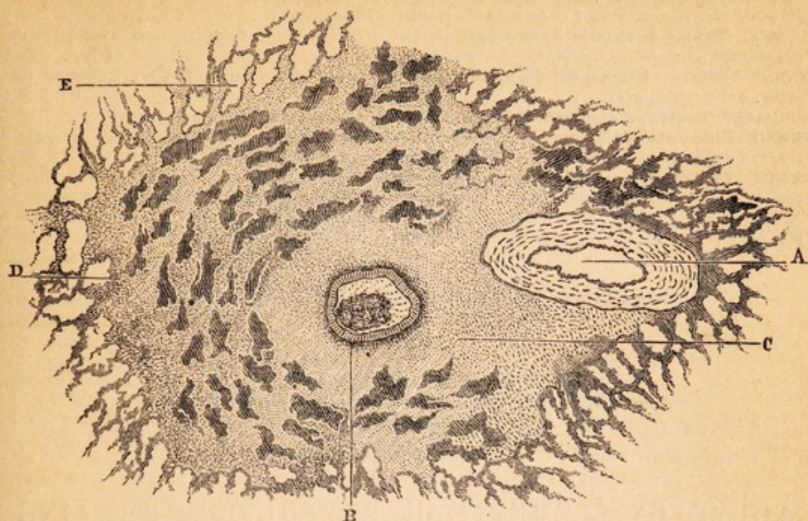
Coupe d'un nodule pérnbronchique.
