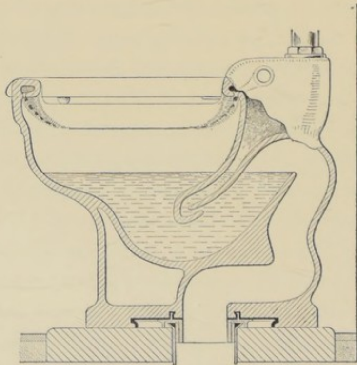
Fig. 25.—Siphon jet closet, "West Point" model (J. L. Mott Co.).
