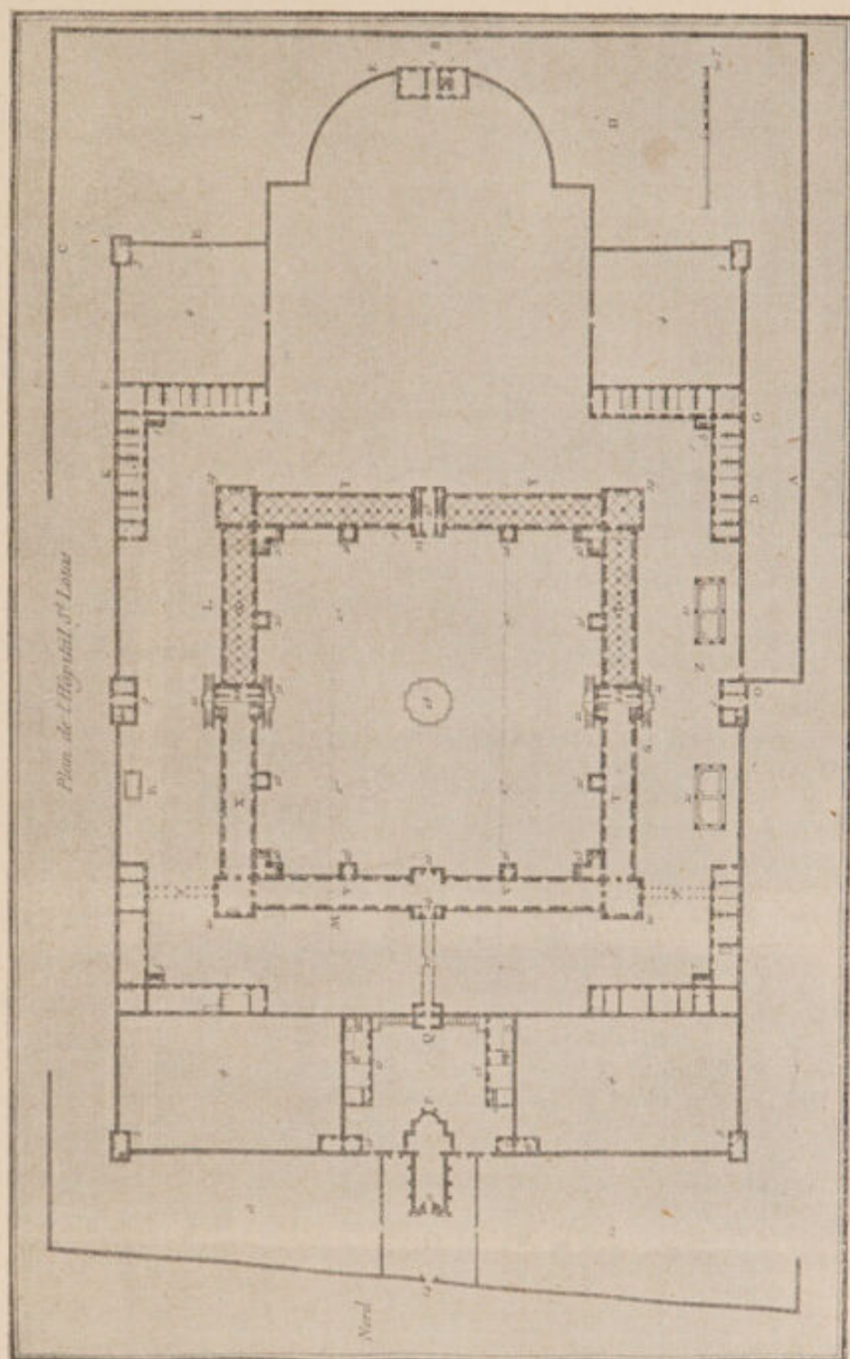
Fig. 8. — Plan de Saint-Louis.
