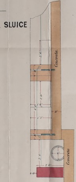
SECTION ON G.H.
