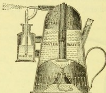
FIG. LXV.—SIEGLE'S ATOMIZER.
