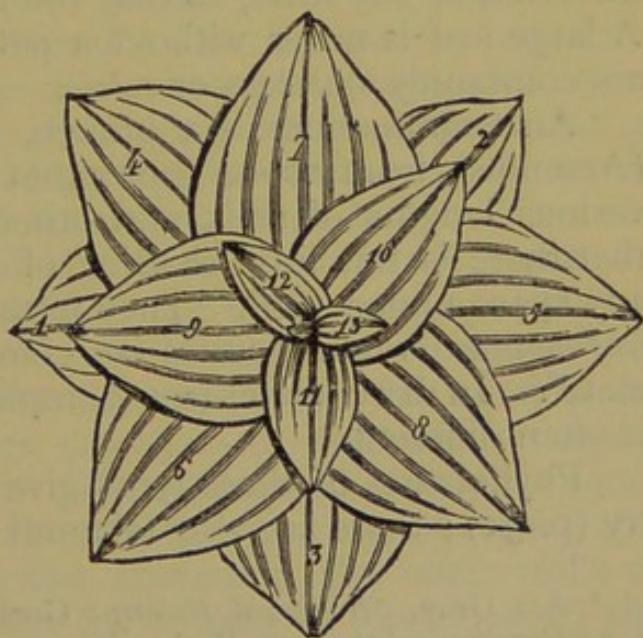
FIG. 2. \frac{3}{8} PHYLLOTAXY.
