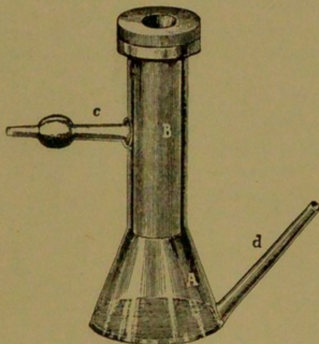
FIG. 11.—Reichel filter.
