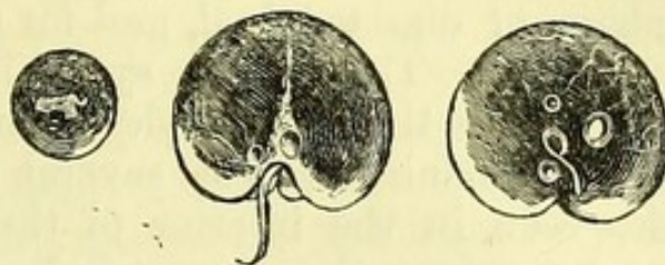
Fig. 217.— Noctiluca miliaris .
