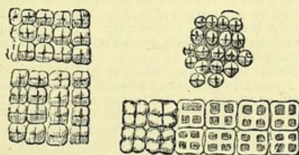
Fig. 158.— Sarcina ventriculi .
