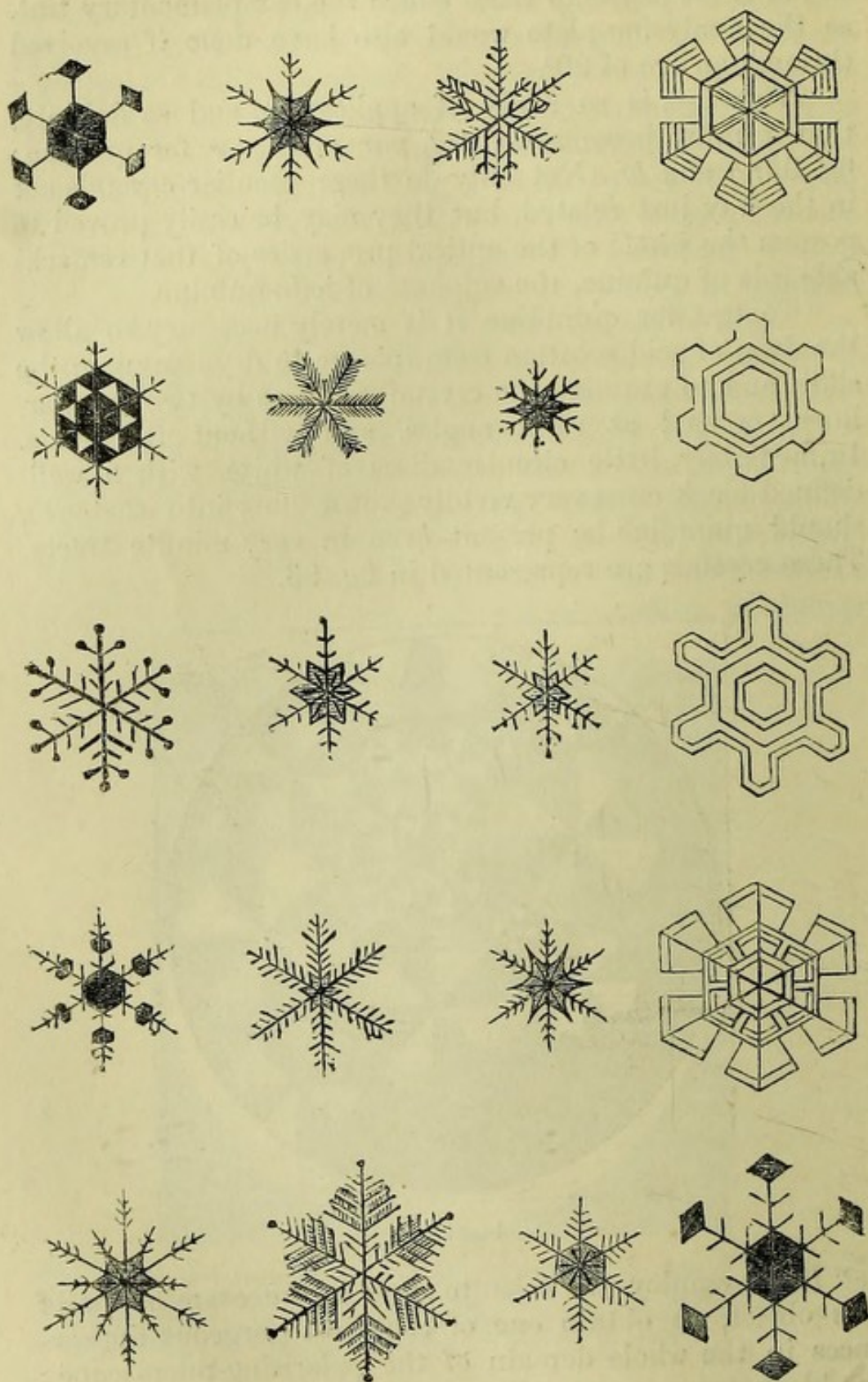
Fig. 94.— Snow Crystals.
