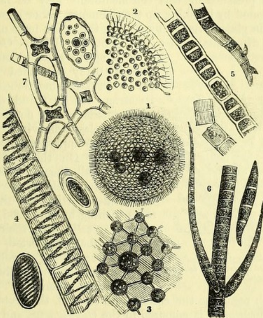
Fig. 145.— Confervæ .
