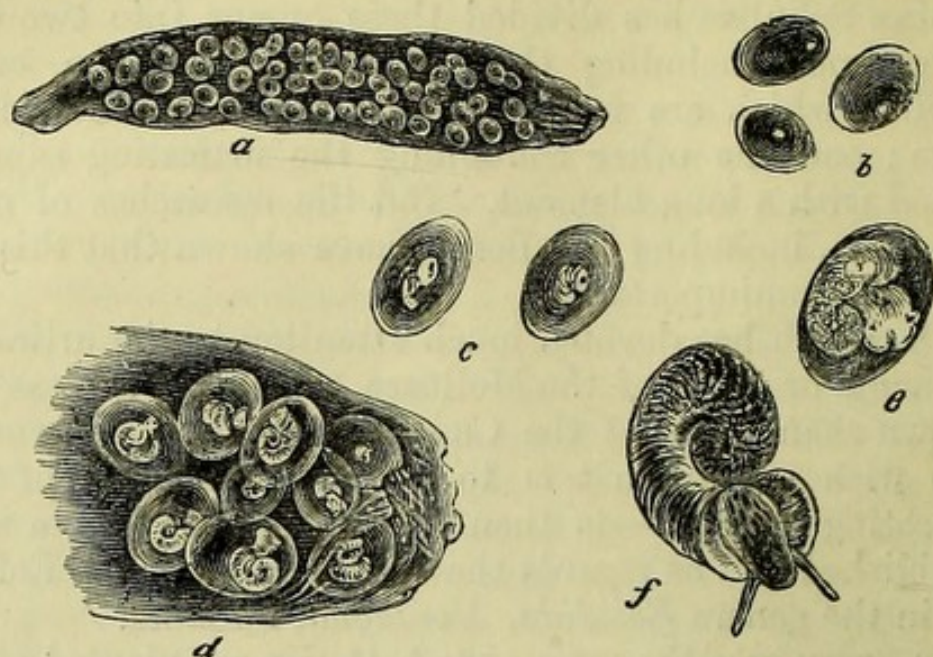
Fig. 252.— Limnæa stagnalis .
