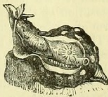
Fig. 248.— Aplysia , sea-hare.
