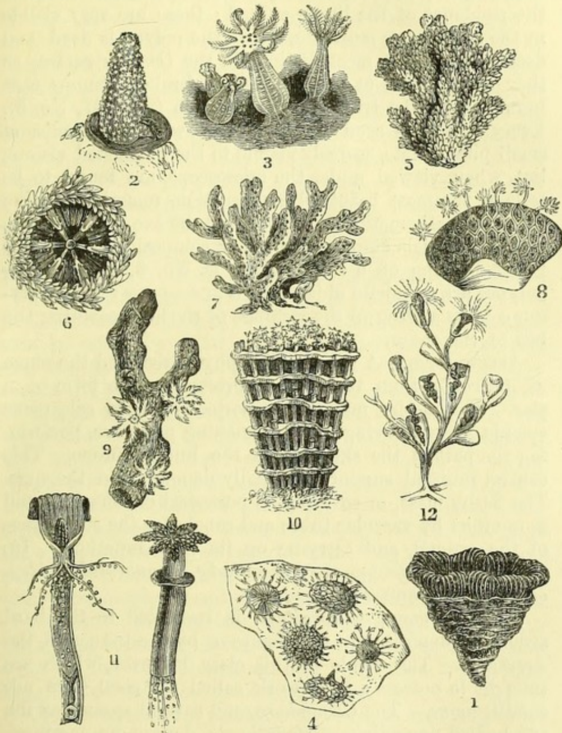
Fig. 237.—Actinozoa.
